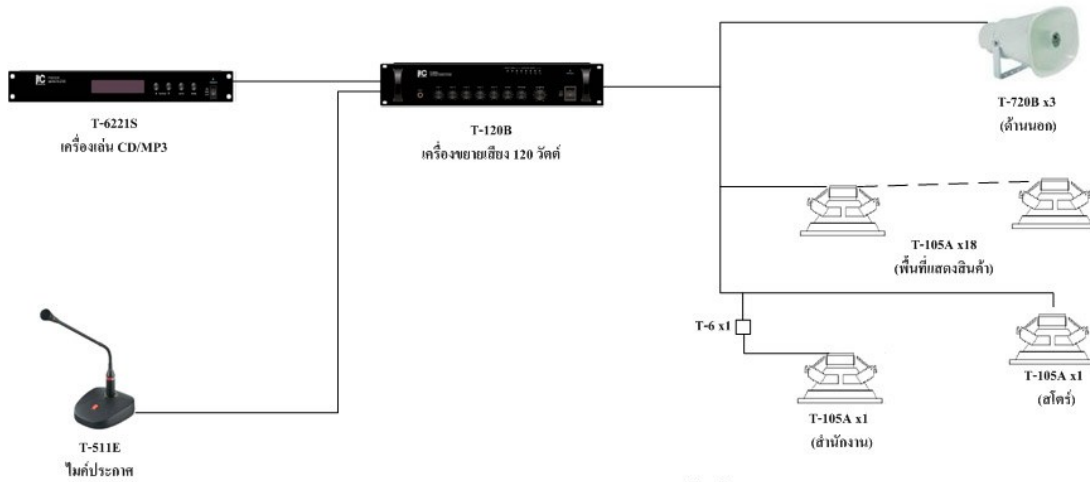
ตัวอย่าง ระบบเสียงสำหรับซูเปอร์มาร์เก็ตชั้นเดียว เช่น Lotus Express
