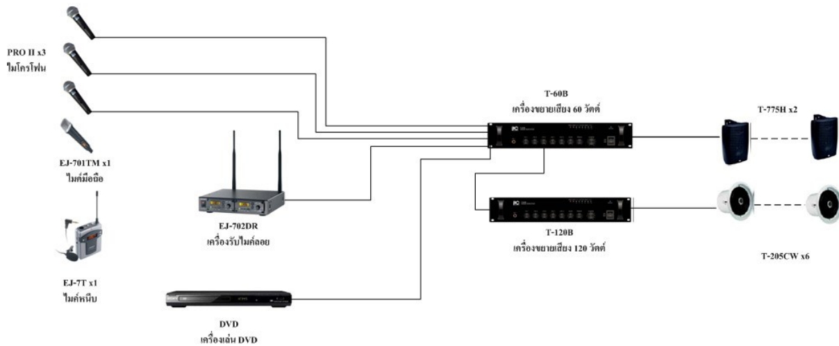
ตัวอย่าง : ระบบเสียงห้องอบรม/ห้องสัมมนา
